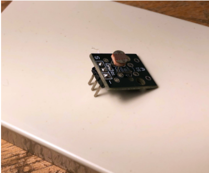
Umgebauter KY-018
