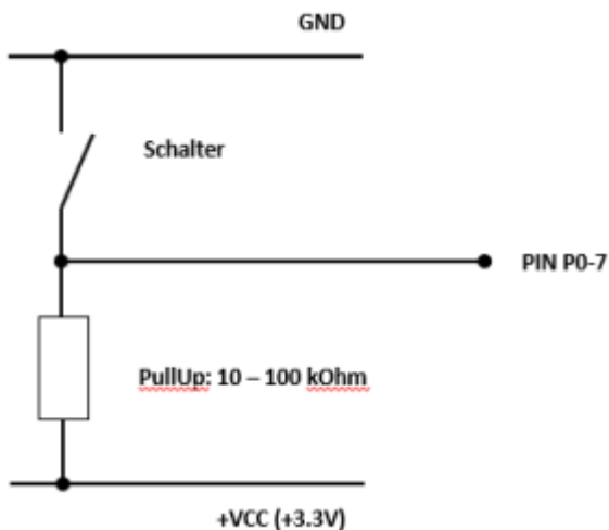
Verschaltung mit externem PullUp-Widerstand
